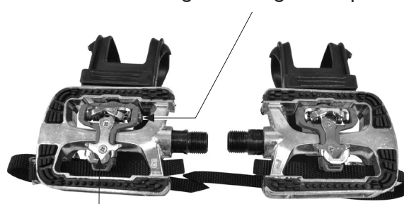
vite di regolazione sgancio rapido
