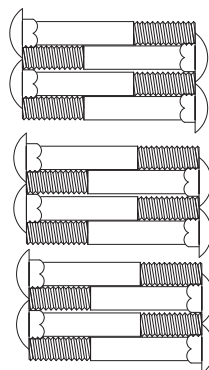
#26 M10×70mm Bullone con quadro sotto testa (12 pz.)
