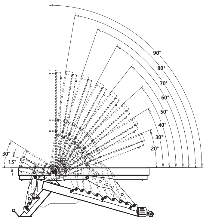
Posizioni di regolazione schienale e sedile
